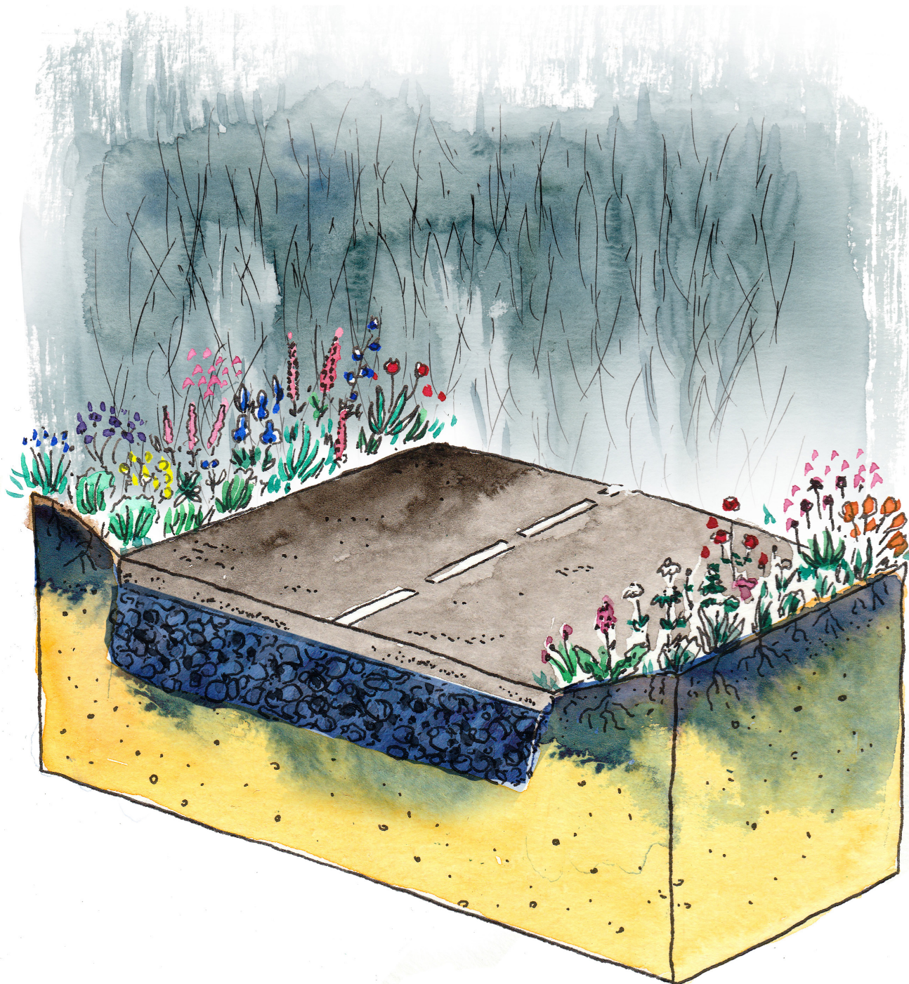
chaussée à structure de réservoir
