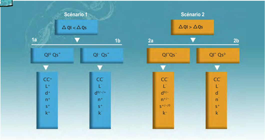
Style d'ajustement du chenal à l'aval d'un barrage en réponse aux modifications relatives des écoulements ( Q_l ) et des entrées de sédiments ( Q_s ), lorsque la métamorphose fluviale est dominée par une réduction de la charge solide, scénario 1, et une réduction des débits, scénario 2. Les conditions extrêmes sont représentées dans les cas 1a et 2b et l'ensemble des configurations (1a, 1b, 2a, 2b) représente des séquences hypothétiques de changements du chenal en aval d'un barrage. À noter cependant que l'importance des modifications du chenal est décroissante vers l'aval ainsi que l'impact du barrage sur les débits liquides et solides. Les indices indiquent l'importance des ajustements : 0, pas de changements significatifs, +, accroissement, - réduction et = réduction majeure. Les variables morphologiques sont : CC-capacité du chenal (c.-à-d. la dimension de la section mouillée), L-largeur, d-profondeur, n-rugosité, s-pente et k-capacité de transport, (d'après Petts et Gurnell, 2005 basé sur Schumm, 1969).
