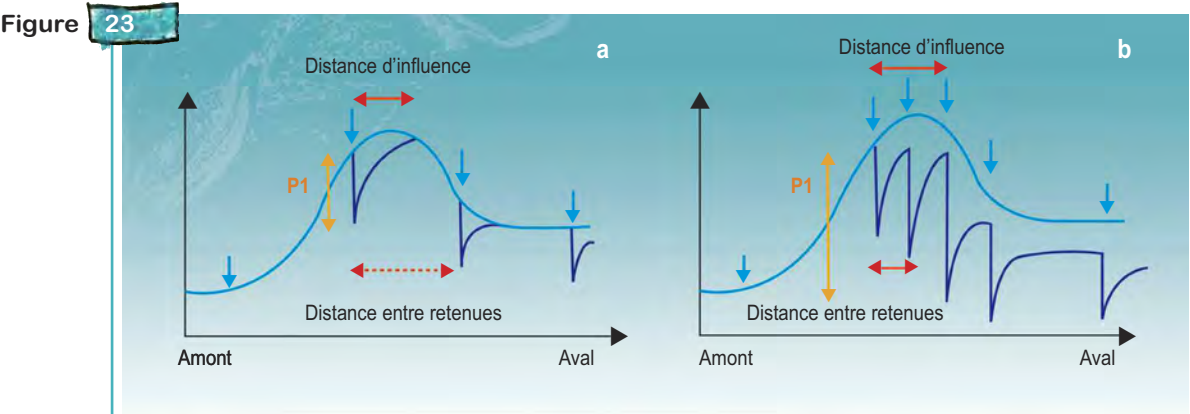
Impact de plans d'eau sur le comportement aval théorique d'une variable, a) sans impacts cumulés, b) avec des impacts cumulés.
