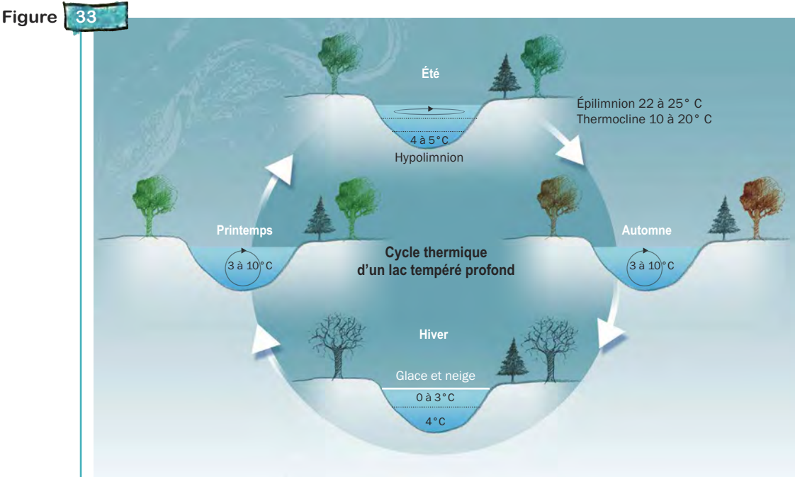
Cycle thermique caractéristique des lacs tempérés dicmitiques (deux périodes de stratification). D'après G Bourbonnais ( http://ici.cegep-ste-foy.qc.ca ).
