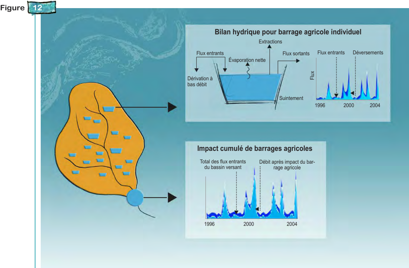
Représentation conceptuelle d'un modèle hydrologique pour la simulation de l'effet cumulé des retenues sur le débit à l'exutoire (modèle TEDI, (Nathan & Lowe 2012)).
