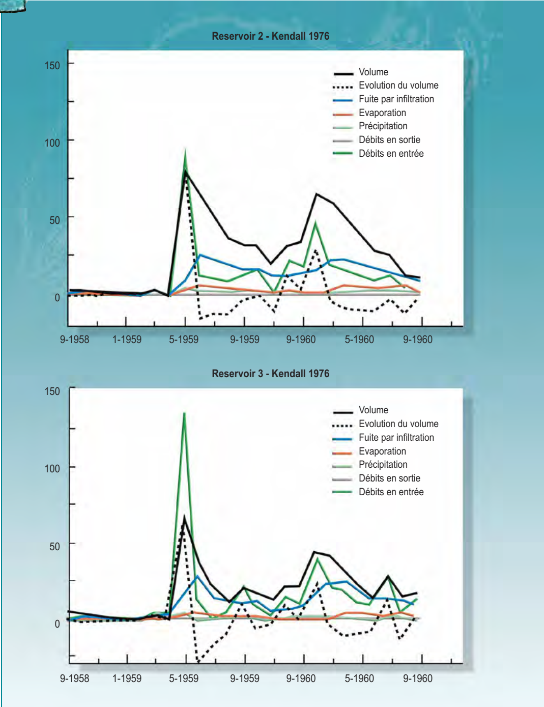
Bilan hydrique mensuel de deux retenues, en Oklahoma, suivies entre septembre 1958 et septembre 1960. Noir : volume de la retenue, noir pointillé : évolution du volume de la retenue, vert foncé : apport sur le bassin d'alimentation, vert clair : précipitation sur la retenue, bleu : perte par infiltration, rouge : perte par évaporation ; gris : débits en sortie. Tous les volumes sont exprimés en milliers de m 3 .
