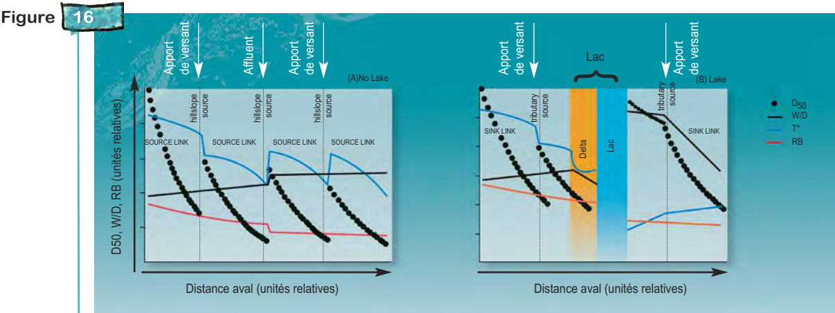
Evolution hydromorphologique le long d'un cours d'eau selon qu'il comporte (B) ou pas (A) un lac (Arp et al., 2007). D50 est la taille médiane des sédiments du lit, W / D est le rapport largeur-profondeur du chenal, T^* est la contrainte de cisaillement sans dimension au débit max pour le D50, et RB est le ruissellement max.
