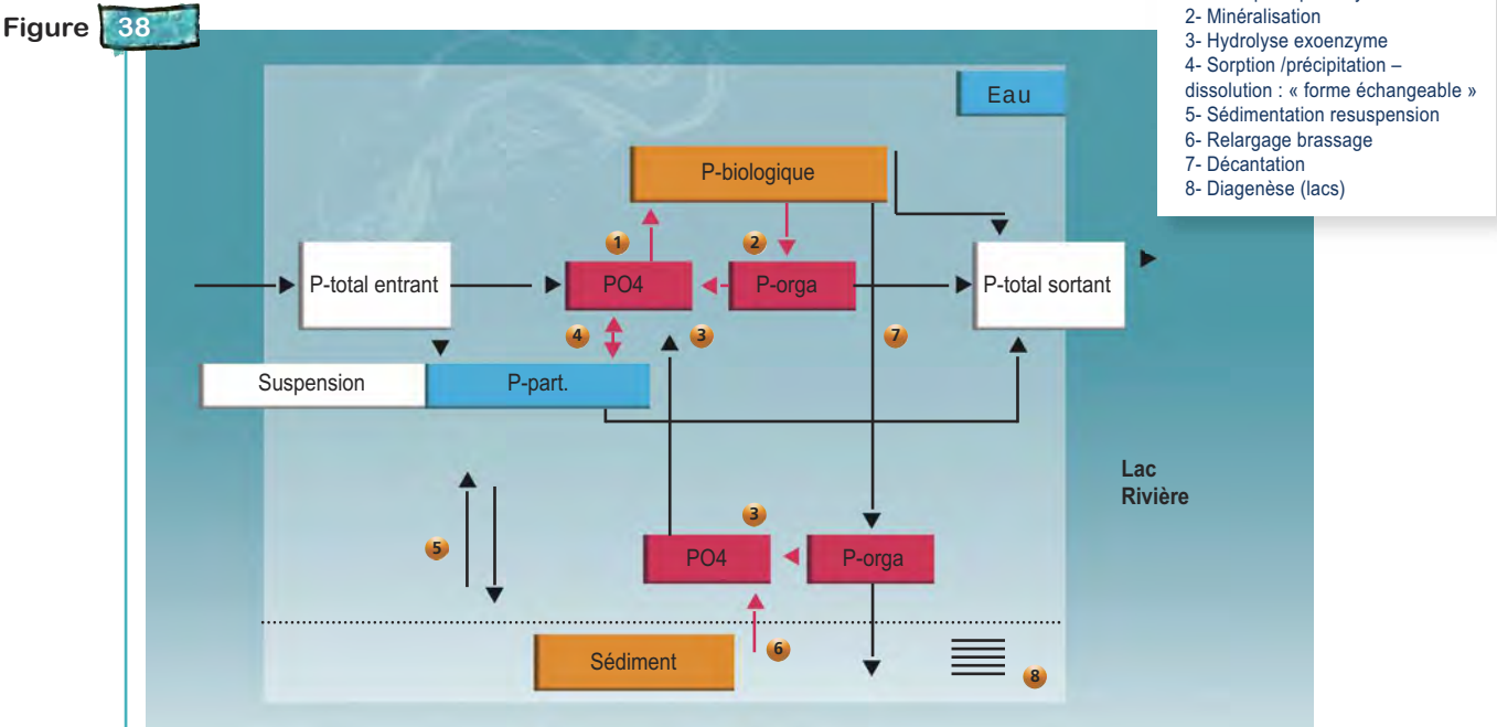
Cycle du phosphore en milieu aquatique : flux, transports et compartiments. D'après traité de limnologie (Pourriot et Meybeck, 1995), modifié.
