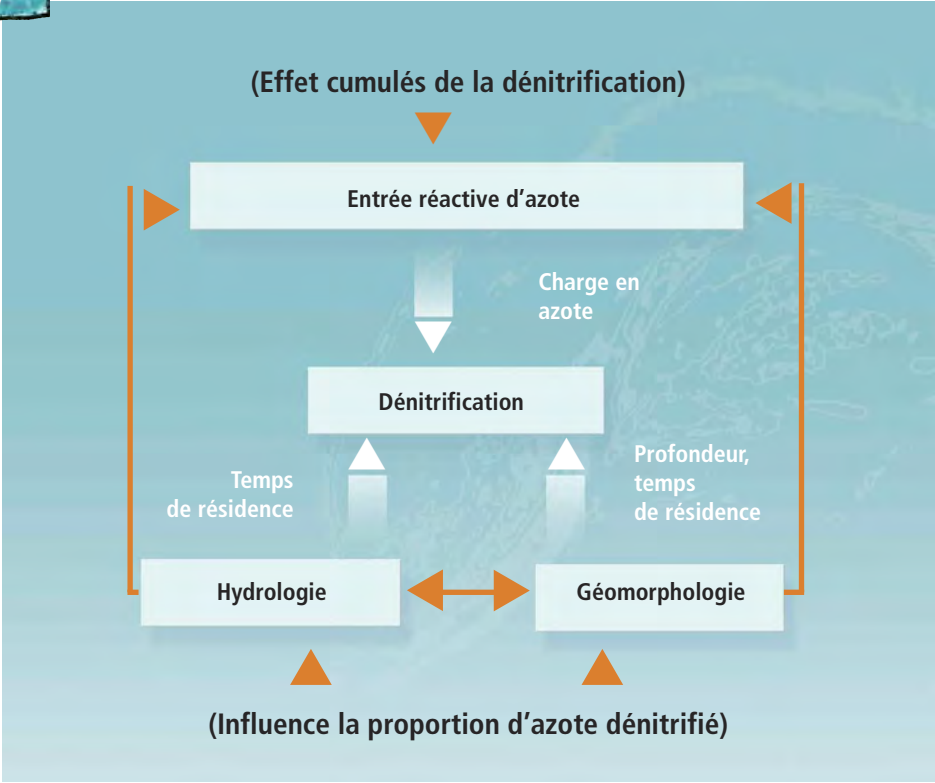
Schéma de l'interaction entre hydrologie, géomorphologie et charge en azote sur la dénitrification. D'après Seitzinger 2006.
