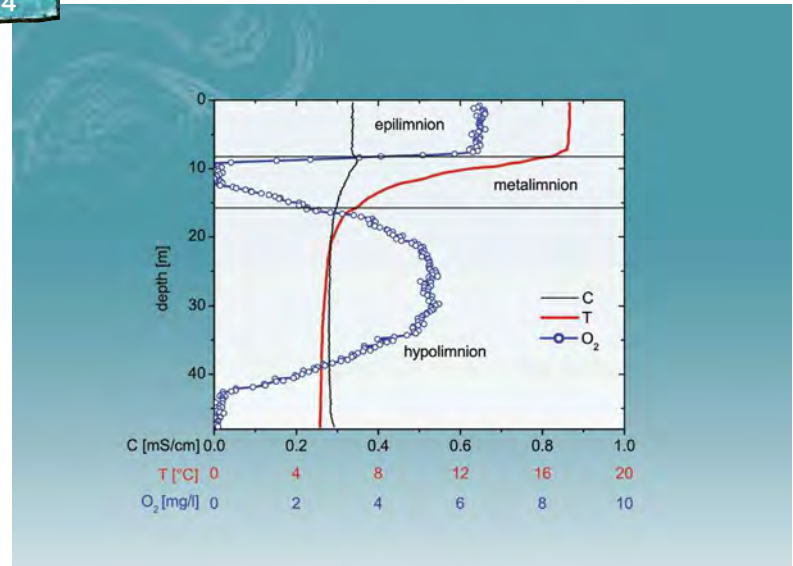
Profil de température (T), de conductivité (C) et de teneur en oxygène dissous (O 2 ) dans le lac Arendsee (Allemagne) le 6 septembre 2000. Boehrer and Schultze 2008.
