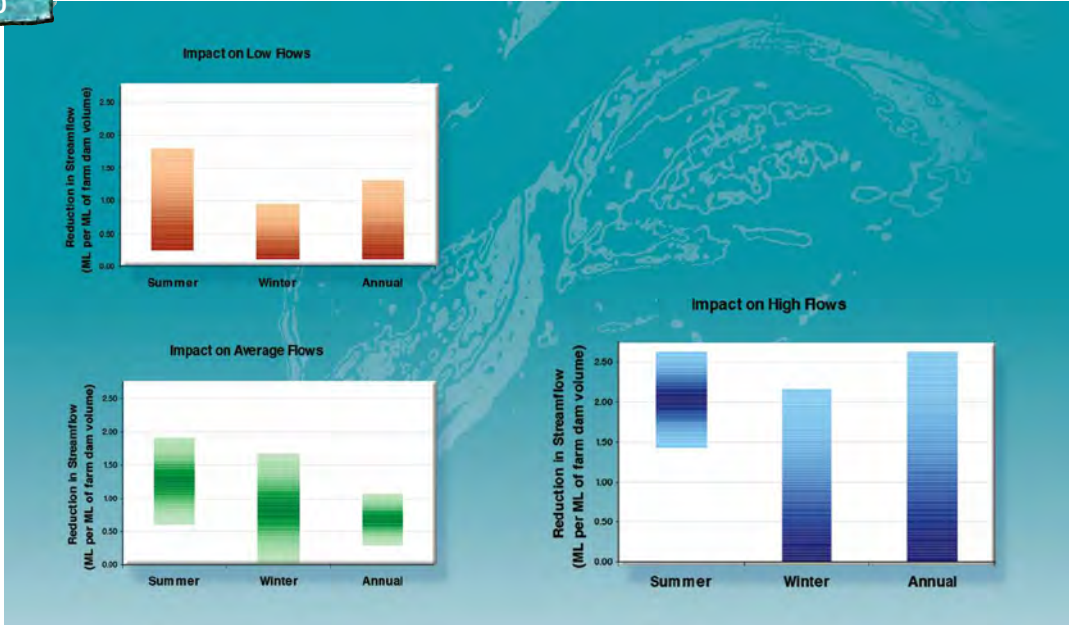
Impacts des réseaux de retenues sur les débits des rivières en été, en hiver et en moyenne sur l'année. La différence de débit est rapportée à la capacité cumulée des retenues. À gauche l'impact sur les faibles débits, au milieu sur les débits moyens et à droite sur les forts débits. Les valeurs sont une compilation d'estimations faites par modélisation sur un ensemble de bassins versants dans la province de Victoria – Australie.
